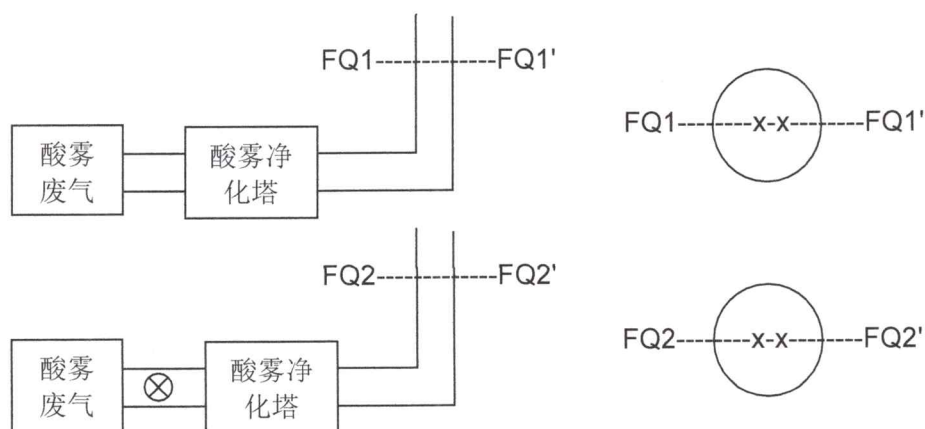
图 2 中国电子科技集团公司第四十四研究所废水检测点示意图
