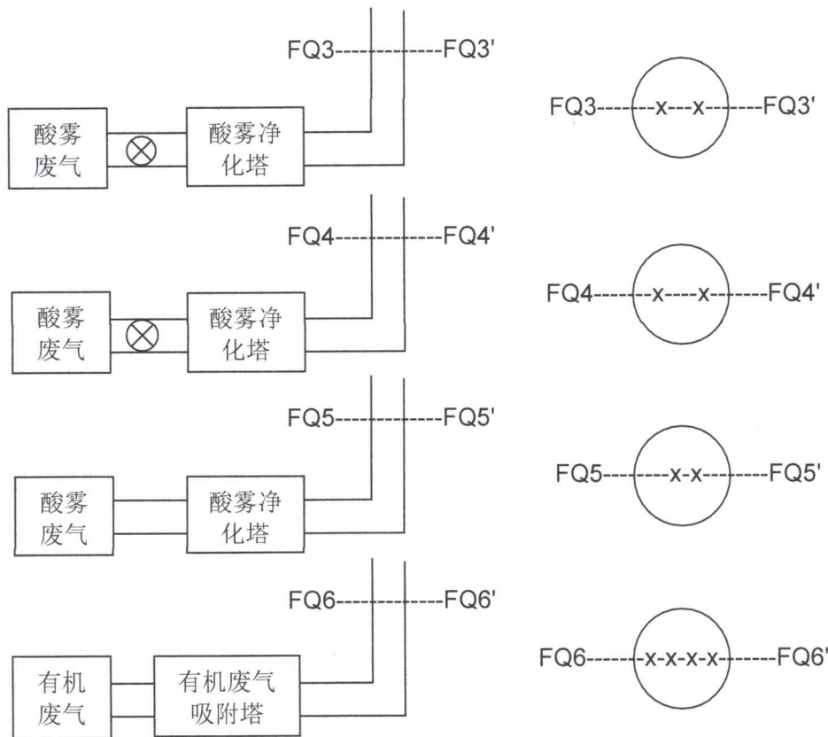
图 3 中国电子科技集团公司第四十四研究所废气有组织检测点示意图
